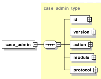
Abbildung 22: Aufbau des Elements <case_admin>
