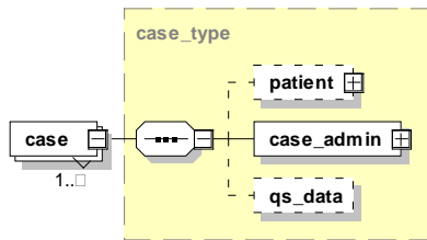
Abbildung 21: Aufbau des Elements <case>
