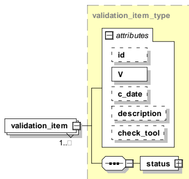
Abbildung 11: Aufbau und Kind-Elemente des Elements &lt;validation_item&gt;
