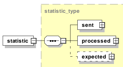
Abbildung 26: Aufbau des Elements <statistic>
