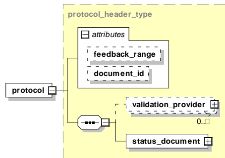
Abbildung 9: Aufbau des Elements <header>/<protocol>
