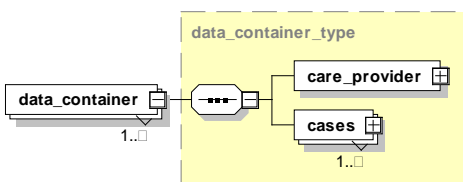
Abbildung 17: Aufbau des Elements <body>/<data_container>
