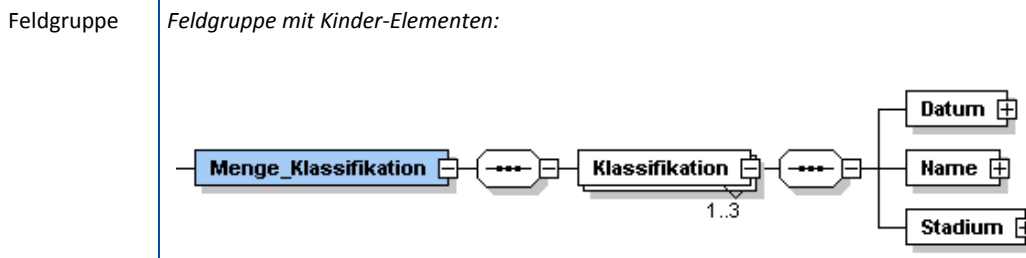
Abbildung 30: Beispiel für den Export einer Feldgruppe
