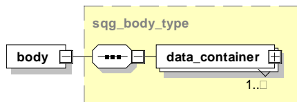
Abbildung 16: Aufbau des Elements <body>
