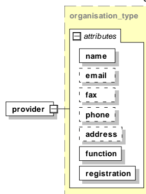
Abbildung 8: Aufbau des Elements <provider>
