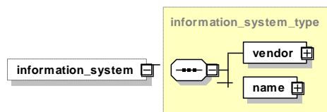
Abbildung 6: Aufbau des Elements <information_system>
