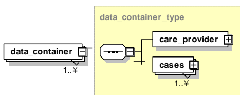
Abbildung 16: Aufbau des Elements <body>/<data_container>
