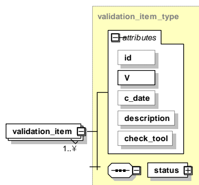
Abbildung 10: Aufbau und Kind-Elemente des Elements &lt;validation_item&gt;
