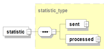
Abbildung 25: Aufbau des Elements <statistic>
