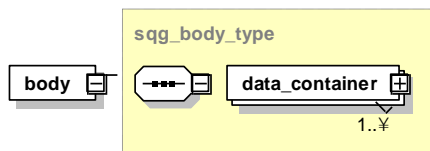
Abbildung 15: Aufbau des Elements <body>
