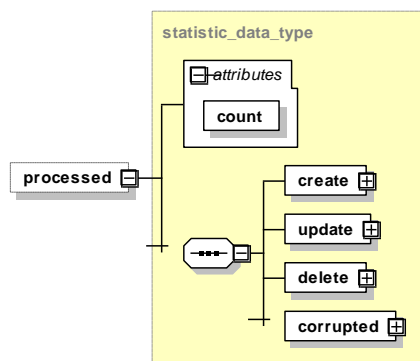
Abbildung 27: Aufbau des Elements <processed>
