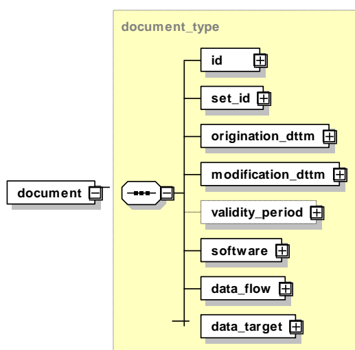
Abbildung 4: Aufbau des Elements <document>
