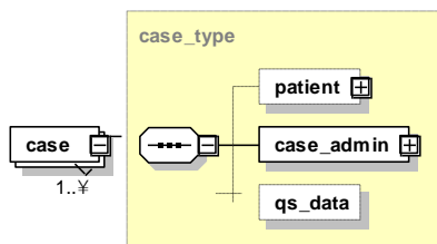
Abbildung 20: Aufbau des Elements <case>
